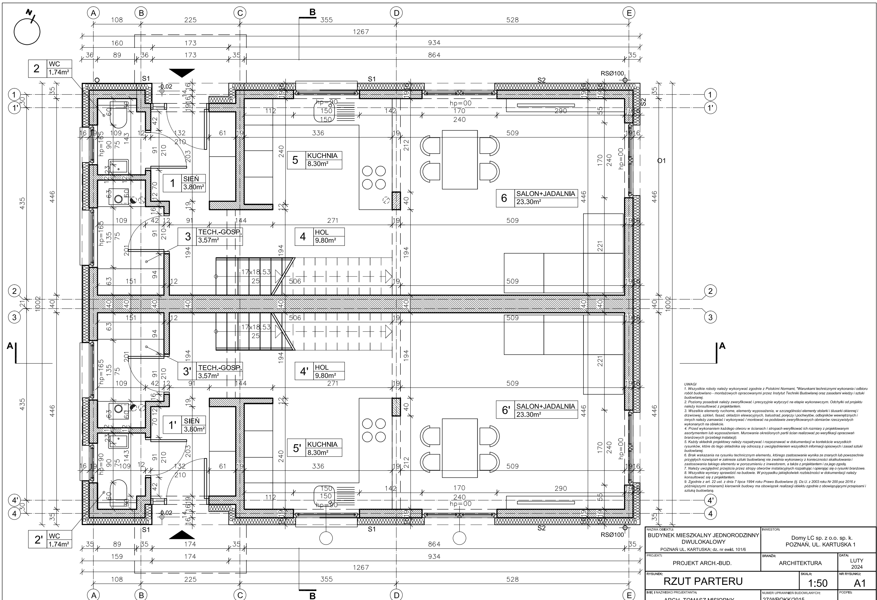
RZUT PARTERU
